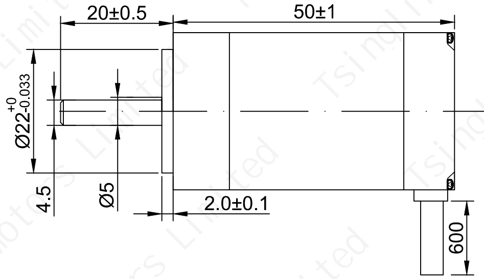
外形尺寸: unit=mm
